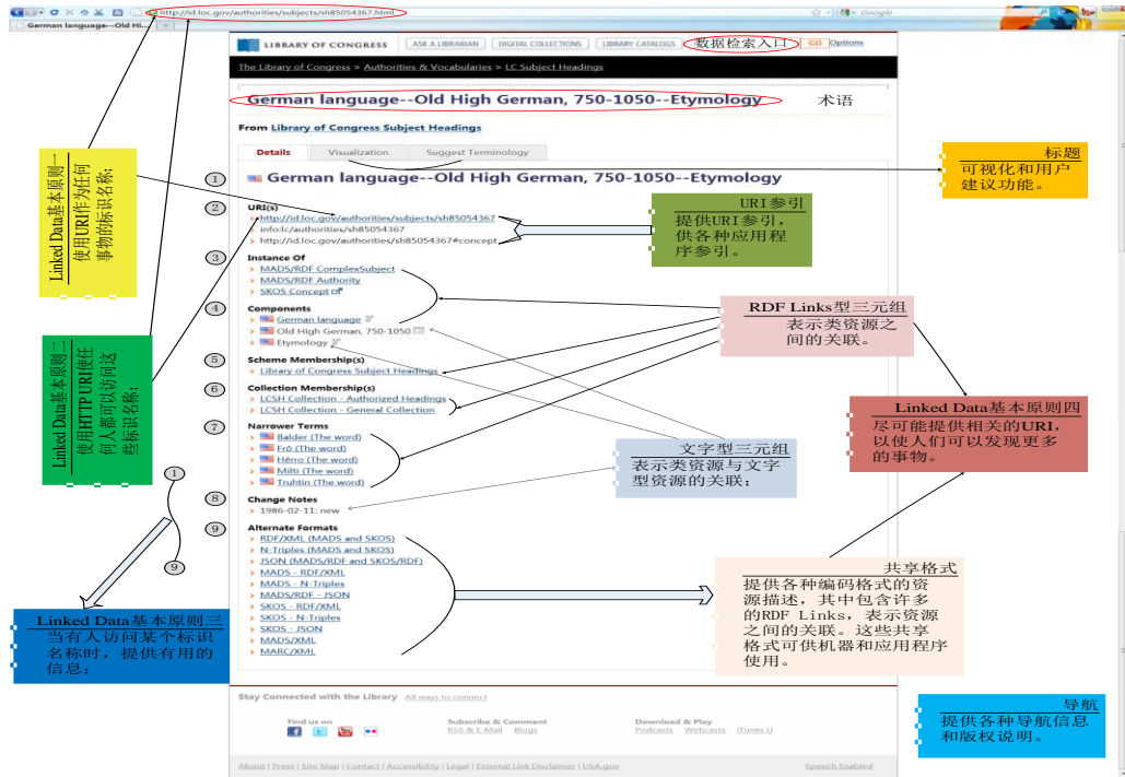
图 2 LCSH Linked Data 服务示意图
