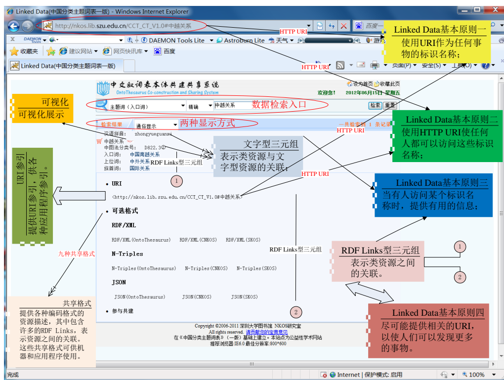
图3 OTCSS Linked Data 服务示意图
